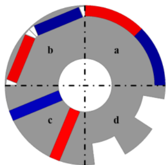
Fig 1. Inner rotor of (a) SPM-CMG, (b) IPM-CMG, (c) FF-CMG and (d) RMG.
